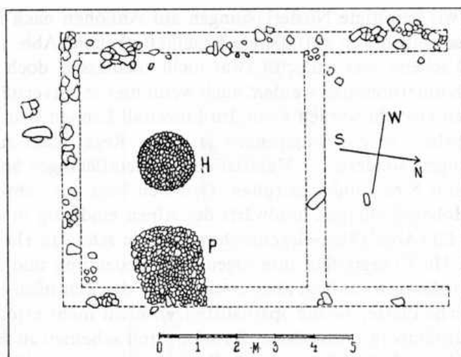
Abb. 17 : Hausgrundriß aus dem Ringwall von Poštela (nach B. Teržan, vgl. Anm. 43, 284 Abb. 22)
