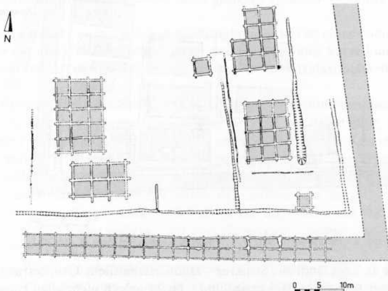
Abb. 1 : Heuneburg IVC (nach W. Kimmig, vgl. Anm. 6, Abb. 33)
